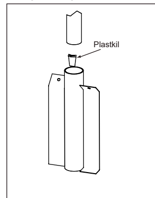
Nedgrävningsfundament 48/76
